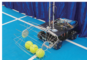
自动捡网球机。
