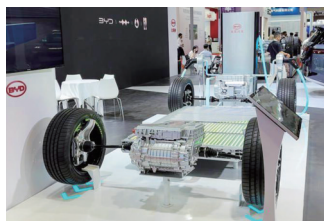
▲比亚迪兆瓦闪充系统
