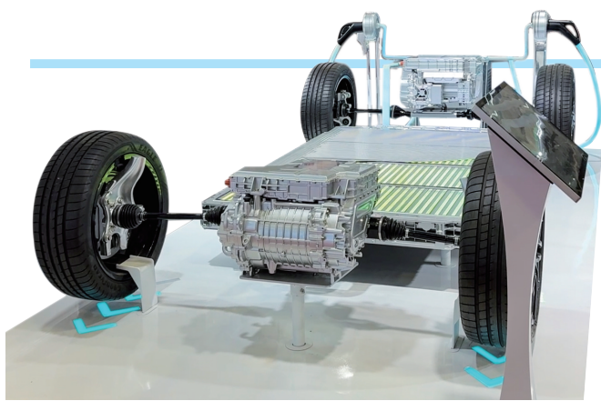
▲比亚迪全球首个兆瓦闪充系统，9分钟可充满电。
